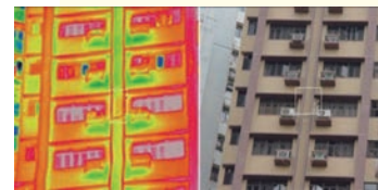
熱紅外技術應用於住房研究
