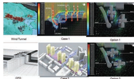
建築群通風環境分析
