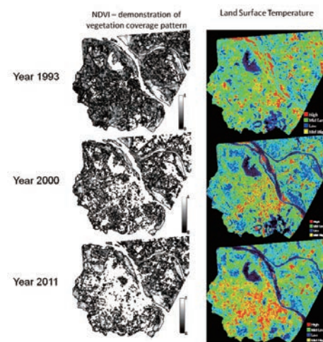
越南河內城市化進程與熱島分布變化關係研究
